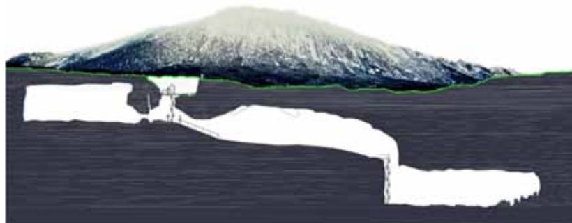
Þversnið af Vatnshelli í Purkhólhrauni. Teikning: Hjörleifur Stefánsson
