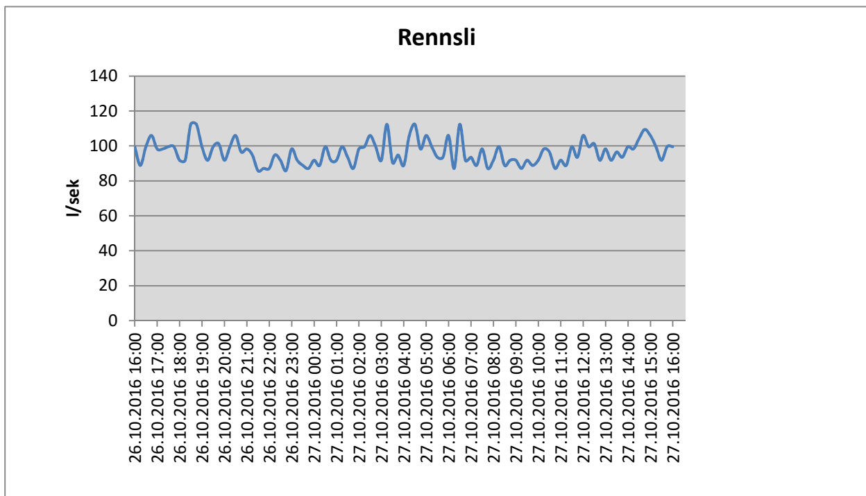
Mynd 2.1.1 Mælt rennsli frá þvottaturnum yfir 24 klst. tímabil
